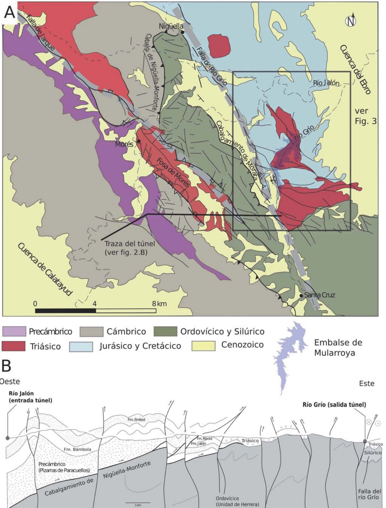
Fig. 2.- A. Mapa geológico del entorno de los ríos Jalón y Grío que indica las principales unidades y fallas. Se muestra también la extensión y trazado de la falla del río Grío, la principal fuente sísmogénica afectada por el embalse de Mularroya (modificado de GEOVEO, IGME, y Casas et al. , 2016). Se ha superpuesto un mapa de fracturación (fallas con desplazamiento) en el entorno del túnel y embalse de Mularroya, realizado a partir de ortofotografías y mapas geológicos. B. Corte geológico a lo largo de la traza del túnel proyectado para el trasvase de agua del río Jalón al embalse de Mularroya.
