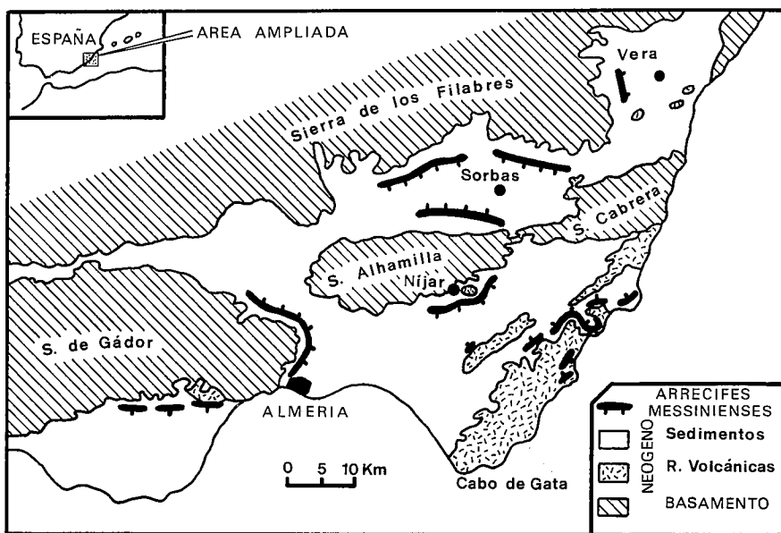
Fig. 1.—Distribución geográfica de los arrecifes messienses en la región de Almería. (Modificada de Dabrio et al. , 1981 y Dabrio et al. , 1985).
