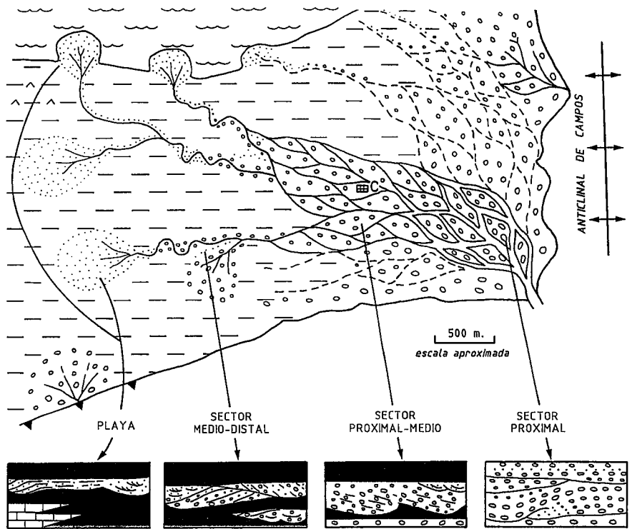
Fig. 2.—Modelo de facies para el abanico superior del sistema aluvial de Cobatillas (UTS A 5 de la cuenca de Aliaga).
