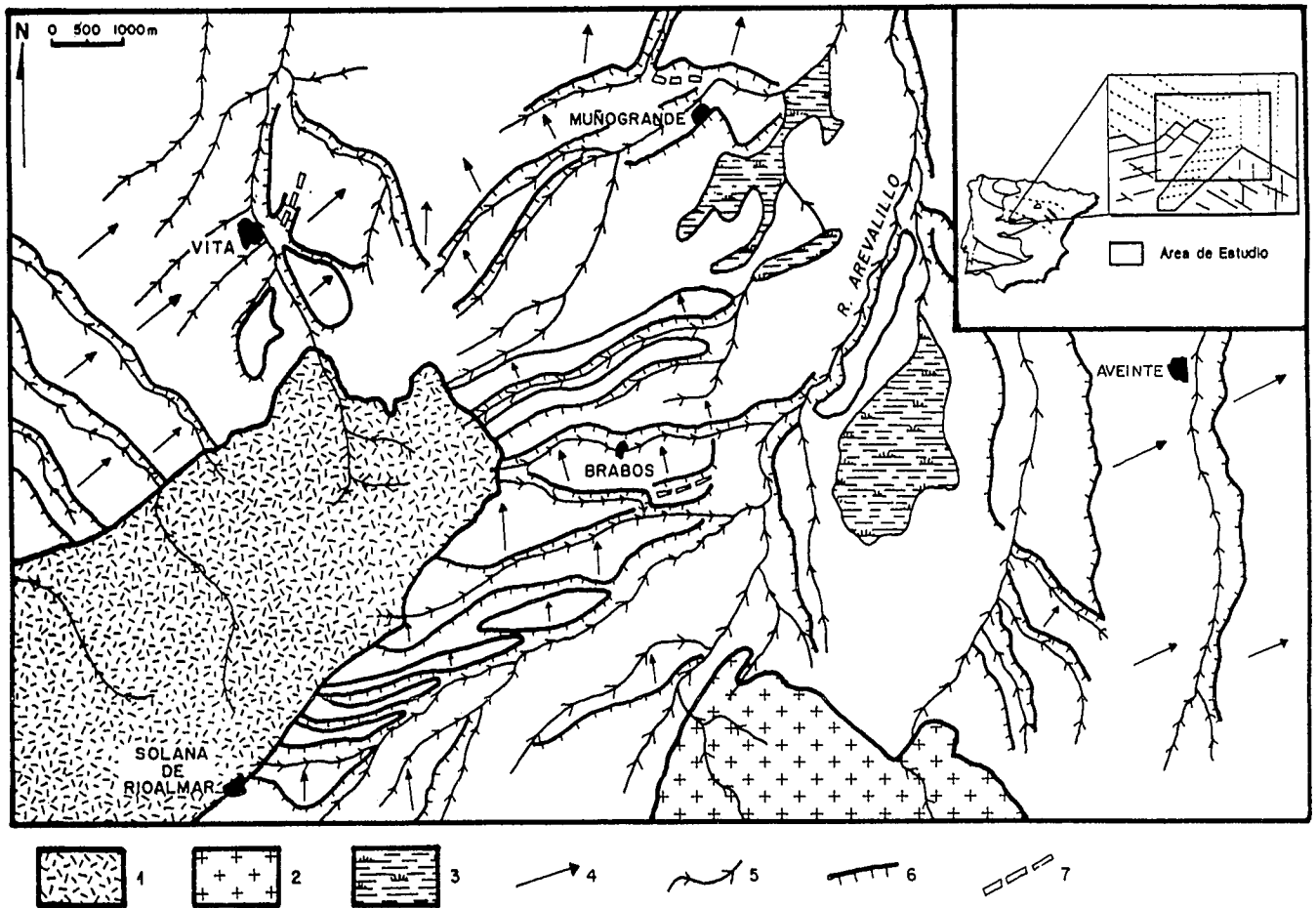
Fig. 1.—Mapa Geomorfológico simplificado del área del Muñico. 1. Zócalo Metamórfico.—2. Zócalo Granítico.—3. Areas deprimidas.—4. Dirección de la vertiente en las cuestas.—5. Cursos fluviales.—6. Escarpe de las cuestas.—7. Cauce abandonado por captura.
