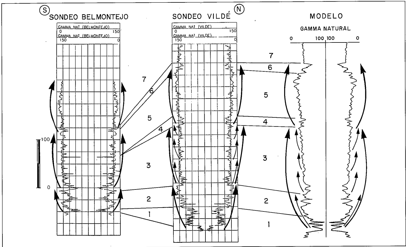
Fig. 2.— Correlación de los sondeos Vildé y Belmontejo con el modelo del Cretácico Superior con diagrañas.
