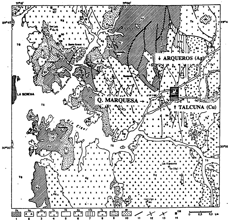
Fig. 1.- Geología de la zona de estudio. 1: Formación Arqueros (Cretácico Inferior); 2: Formación Quebrada Marquesa (Cretácico Inferior); 3: Formación Viñita (Cretácico Superior); Formación Los Elquinos (Terciario Inferior); 5) Rocas sedimentarias (Mioceno -Cuaternario); 6) Granitoides del Cretácico Inferior-Superior; 7) Intrusivos andesíticos y basálticos (Cretácico Superior -Terciario Inferior); 8) Granitoides (Terciario Inferior); 9) Rocas córneas; 10) Zonas de alteración hidrotermal; 11) Fallas; 12) Anticlinal; 13) Sinclinal; 14) Datación K/Ar. Boric (1985).
