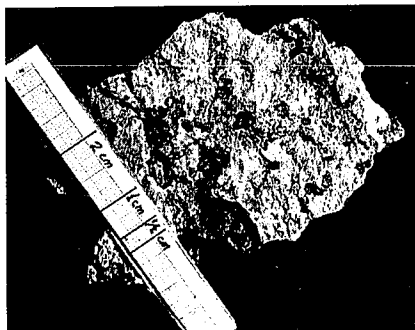
Fig. 6.- Aspecto en muestra de mano de segundo tipo de nódulos. Estos nódulos son de mayor tamaño y de morfología más irregular que los nódulos micríticos de la Fig. 2 y su textura inicial no se conserva.
