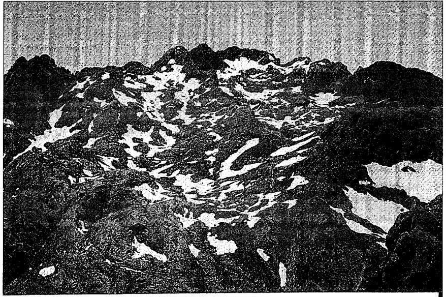
Fig. 2.- Vista de la cara noreste de la Torre del Llambrión, en el Macizo Central de los Picos de Europa. Por ella discurre el itinerario seguido por Casiano de Prado en 1856.
