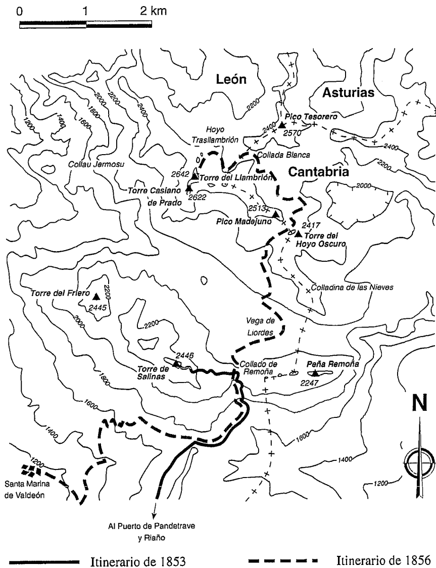
Fig. 1.- Recorrido probable de Casiano de Prado en la ascensión a la Torre de Salinas (año 1853) y a la Torre del Llambrión (año 1856).
