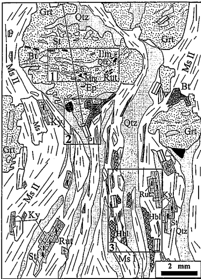
Fig. 2- Esquema textural de la muestra SPP-882 en el que se muestran los microdominios en los que se han realizado determinaciones geotermométricas
