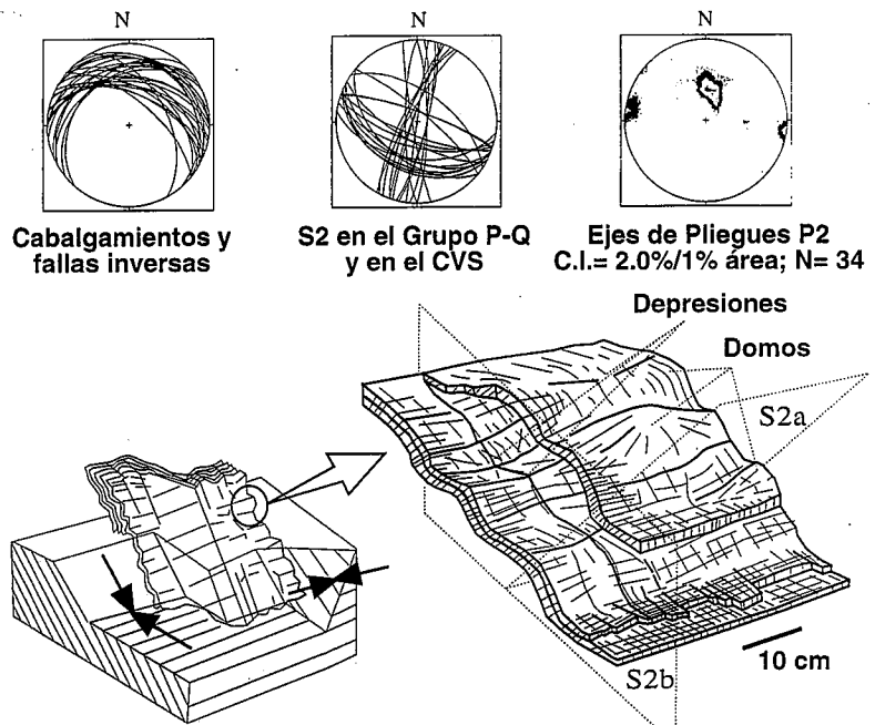
Figura 3. Orientaciones de las superficies de cabalgamiento, foliaciones S2a y S2b y diagrama de densidad para los ejes de pliegues P2a y P2b -proyecciones equiares realizadas en el hemisferio inferior-. Esquema de pliegues tipo domos-cubetas y su relación con los cabalgamientos.
