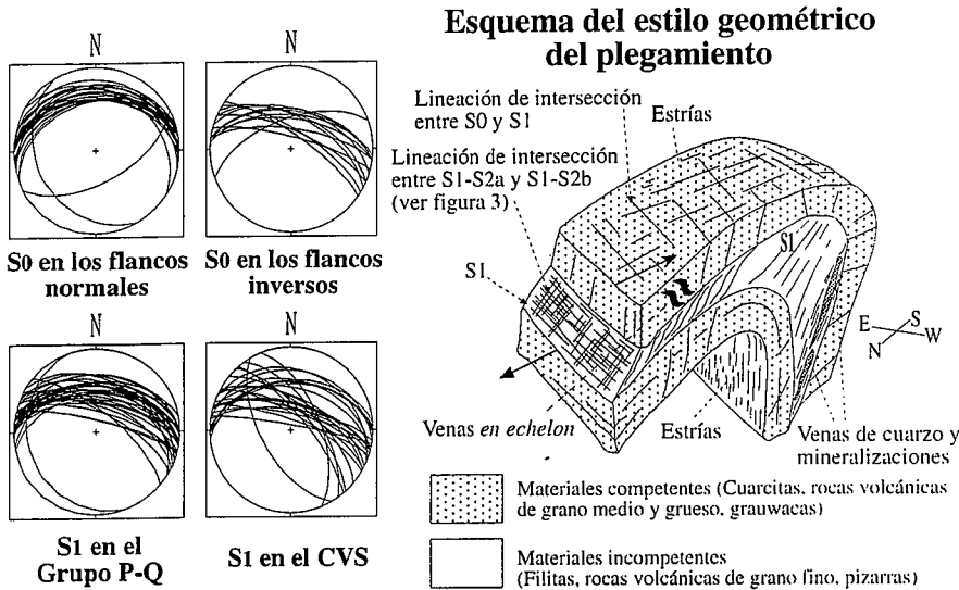
Figura 2. Datos estructurales relacionados con los pliegues cerrados (P1) -Proyecciones equiares realizadas en el hemisferio inferior-. Esquema geométrico de los pliegues y estructuras asociadas.
