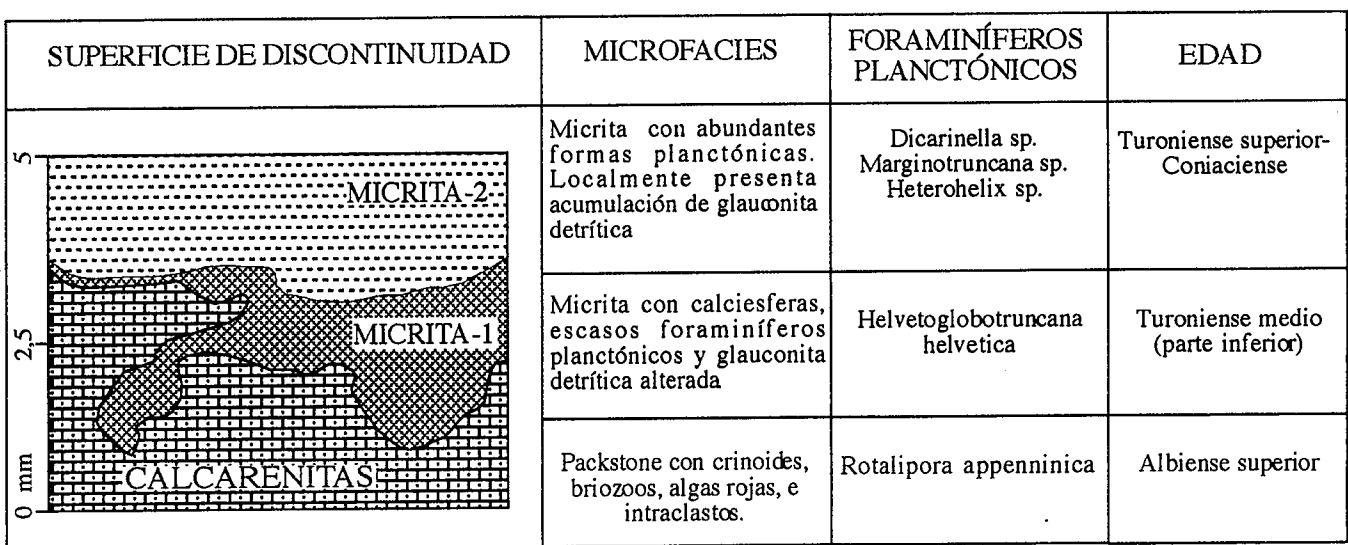
Fig. 3: Esquema de la superficie de discontinuidad con las microfacies observadas: calcarenita basal y dos tapices micríticos.
