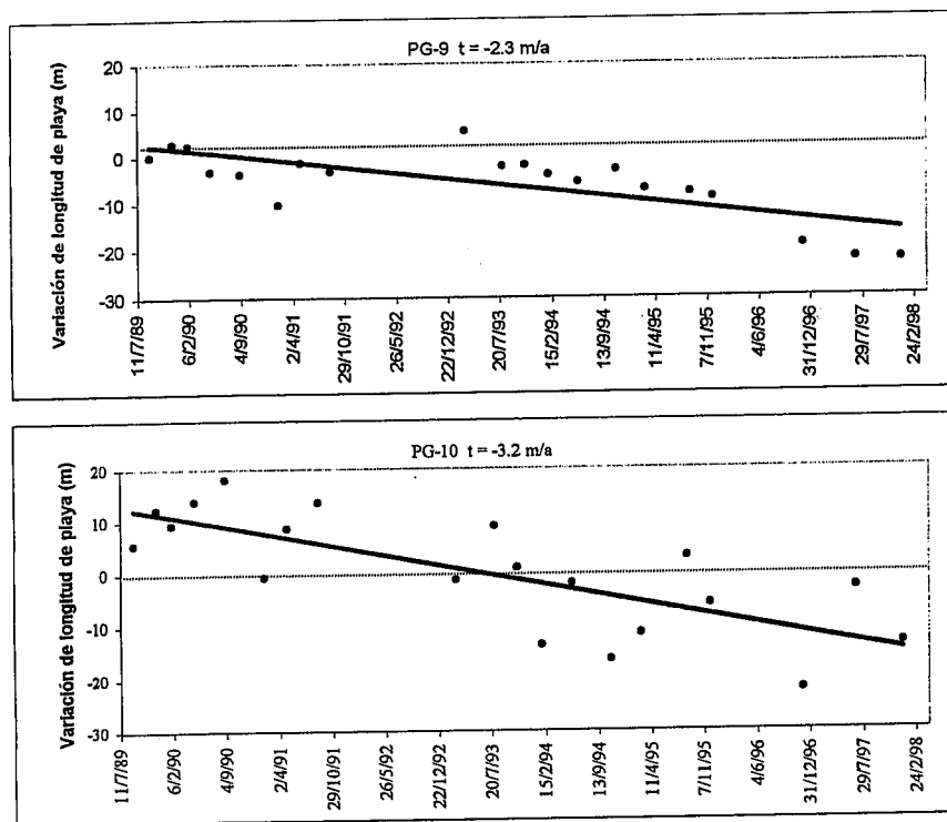
Fig. 4: Variaciones de la longitud de playa en el sector de Vilassar para los perfiles PG-9 (a) y PG-10 (b)
