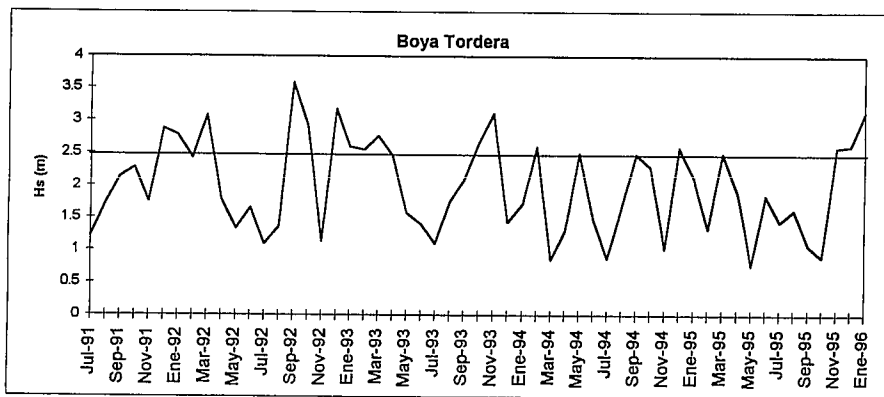
Fig 2: Variación de la altura significativa (Hs) máxima mensual registrada en la boya del Tordera para el periodo 1986-1996.
