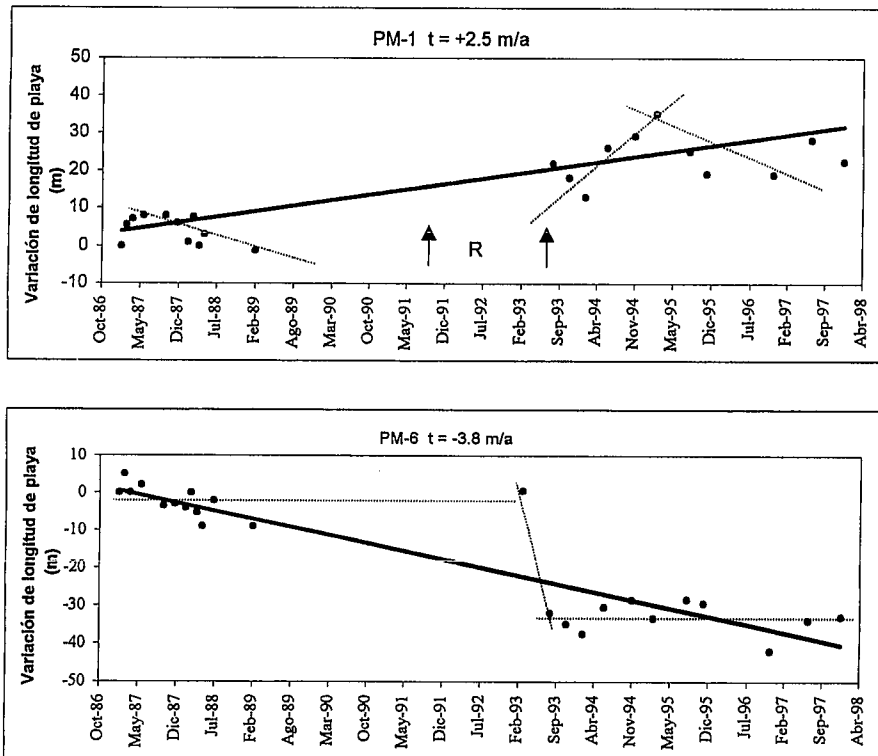
Fig. 3: Variaciones de la longitud de playa en el sector de Malgrat para los perfiles PM-1 (a) y PM-6 (b)
