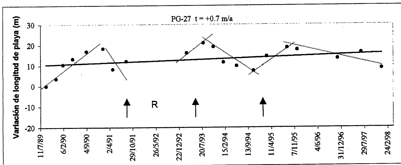
Fig. 5: Variaciones de la longitud de playa en el sector de Masnou-Mongat para el perfil PG-27.
