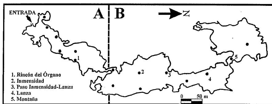
Fig. 1.- Planta de la Cueva de Nerja, localización de los goteros en los que se han hecho medidas y referencia de los considerados en el presente estudio. A: Galerías Turísticas, B: Galerías Altas.
