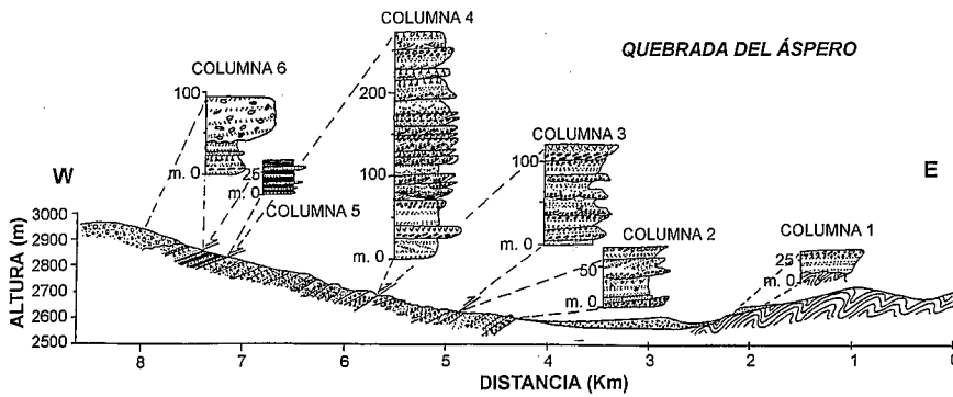
Fig. 2.- Perfil geológico del área de estudio y columnas estratigráficas levantadas.
