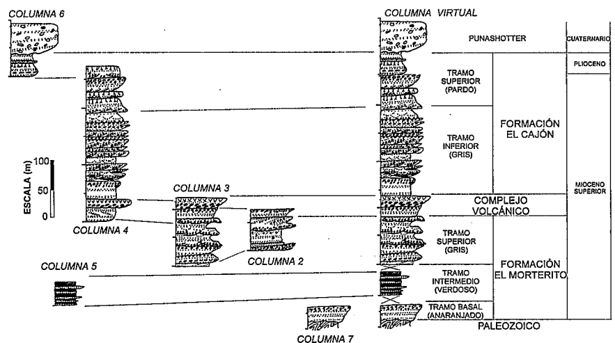
Fig. 3.- Columna estratigráfica tipo del Valle del Cajón.
