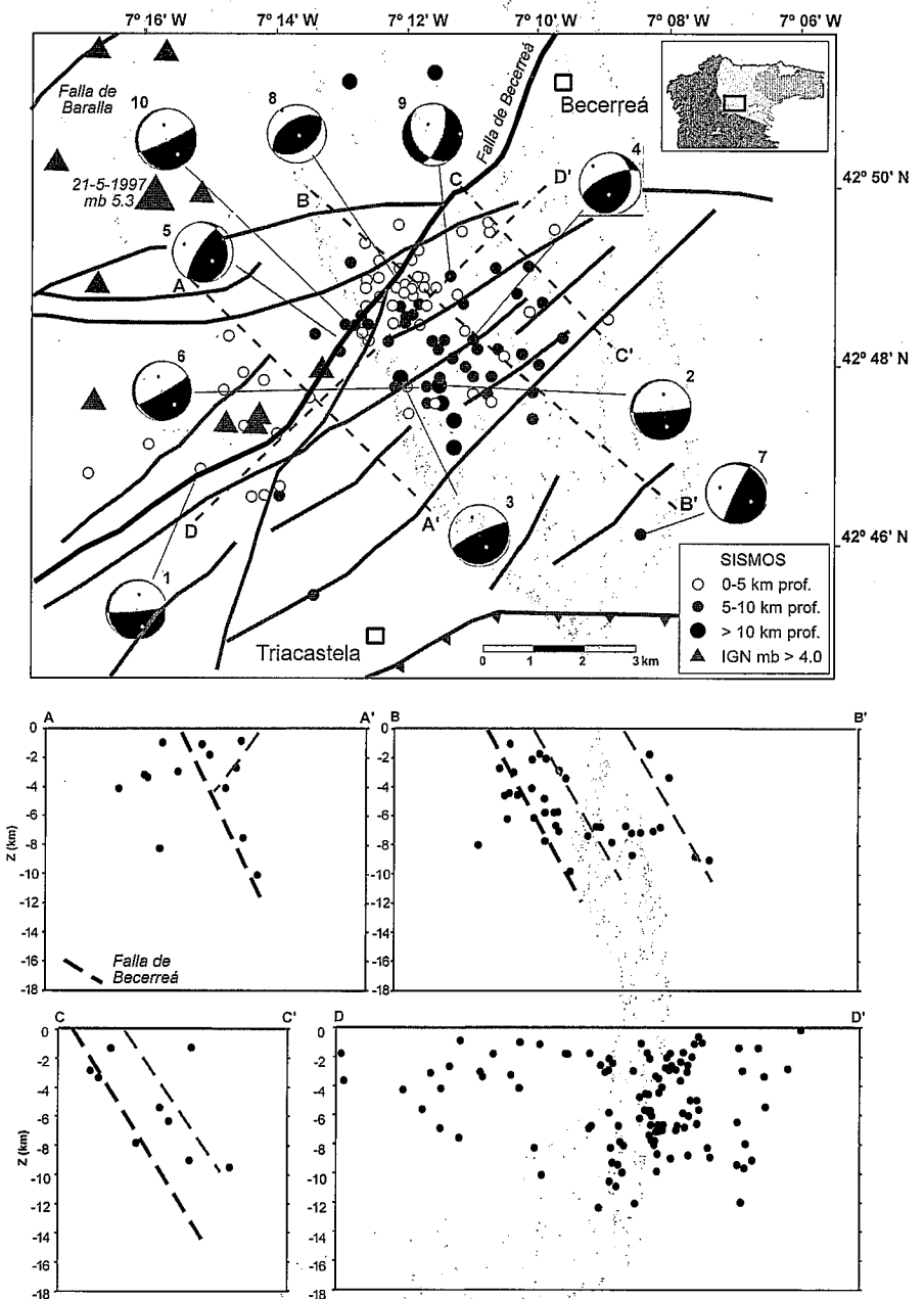
Fig. 4.- (a) Selección de sismos con alta precisión en su determinación hipocentral. Distribución en profundidad de la actividad a lo largo de (b, c, d) perfiles transversales a las principales estructuras y (d) según un perfil longitudinal a la Falla de Becerreá.
