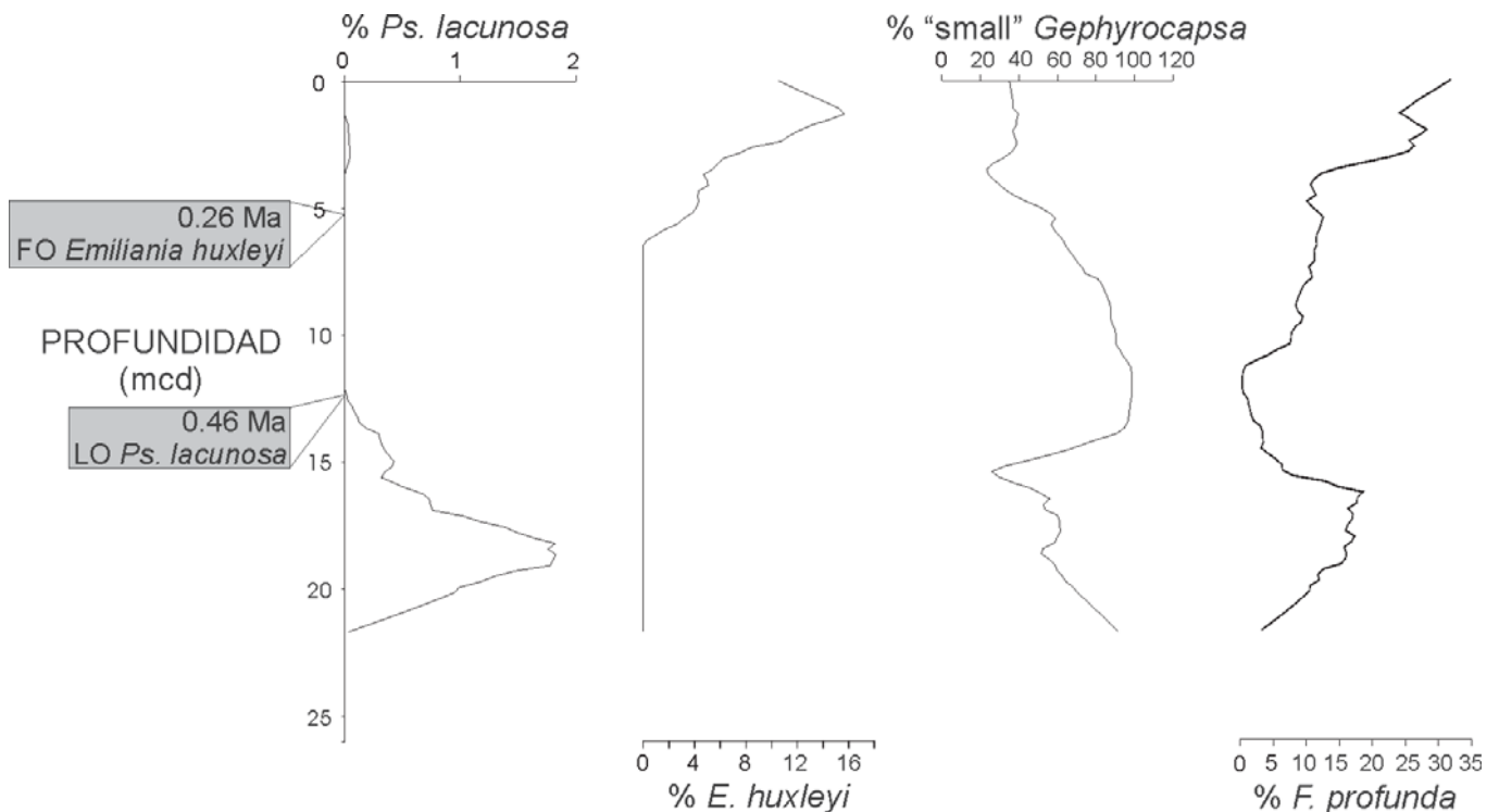
Fig. 3.- Abundancia relativa de varias especies de Cocolitofóridos identificadas en el testigo ODP 1237. Se indica la profundidad de los eventos bioestratigráficos empleados para la elaboración del modelo de edad. FO: primer registro; L.O: último registro; mcd: metros de profundidad compuesta.
