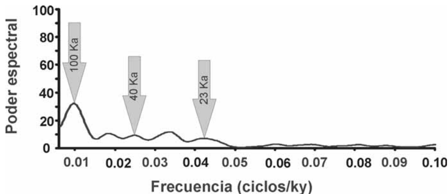
Fig. 2.- Periodograma de los porcentajes de Florisphaera profunda en el testigo ODP 1237 (programa empleado «Analyseries» 1.1., Paillard et al. , 1996).
