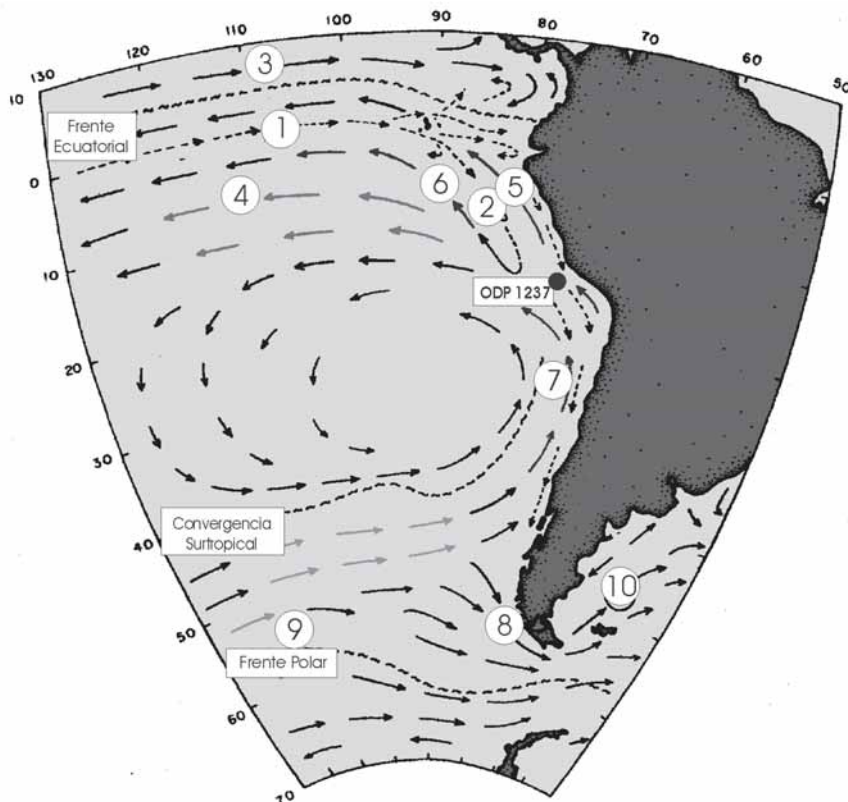
Fig. 1.- Situación del testigo ODP 1237 y representación de los principales rasgos oceanográficos superficiales en la región: Corriente Circumpolar Antártica 9, sistema de corrientes de Peru-Chile (corriente de Chile 7 y sistema de corrientes de Peru: corriente costera de Perú o corriente de Humboldt 5 y corriente oceánica de Peru 6), y corriente Surecuatorial 4. Otras corrientes superficiales, subsuperficiales y contracorrientes en el SE del Pacífico: corriente Subsuperficial Ecuatorial 1, contracorriente de Peru 2, contracorriente Norecuatorial 3, corriente del Cabo de Hornos 8 y corriente de Falkland 10. Modificado de: Molina-Cruz y Herguera (2002).
