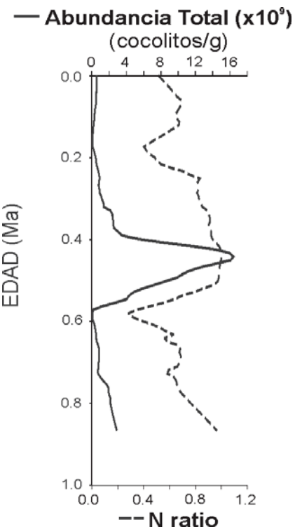
Fig. 4.- Abundancia total de cocolitos y variaciones del índice N vs. edad en el testigo ODP 1237 (ver texto para su definición e interpretación).
