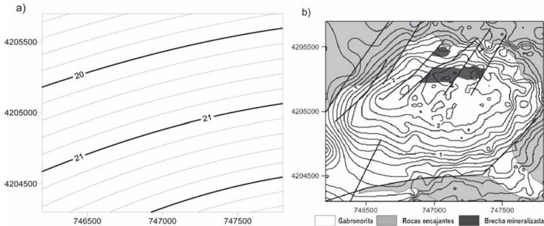
Fig. 4.- a) Mapa de anomalías regionales. b) Mapa de anomalías residuales sobre el que se ha superpuesto el esquema geológico. La gabronorita de Aguablanca está asociada al máximo gravimétrico. En ambos mapas el intervalo entre isoanómalas de 0.2 mGal. Coordenadas UTM, 29 en metros.
