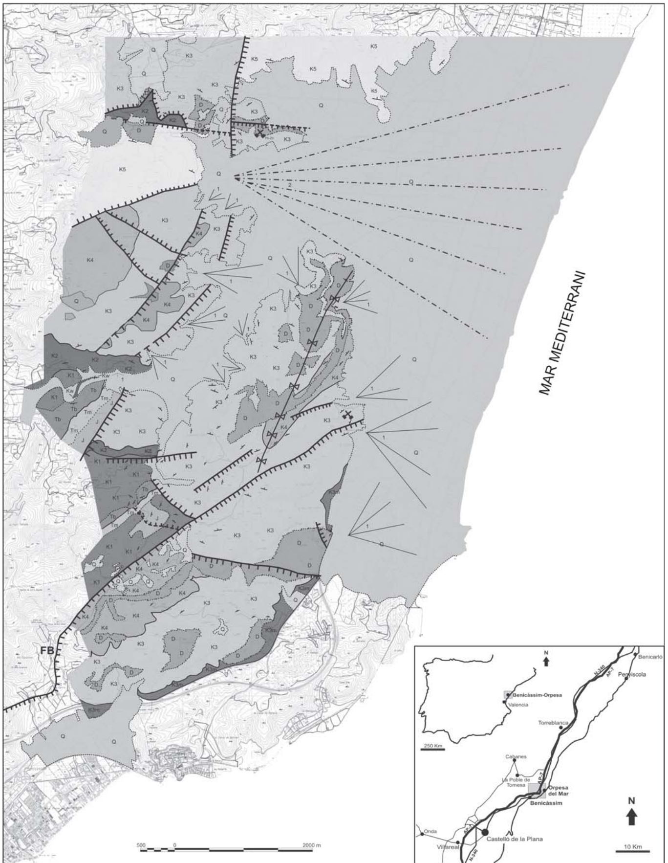
Fig. 1.- Mapa geològic de la zona de Benicàssim-Orpesa, donde se indica la falla de Benicàssim (FB).
