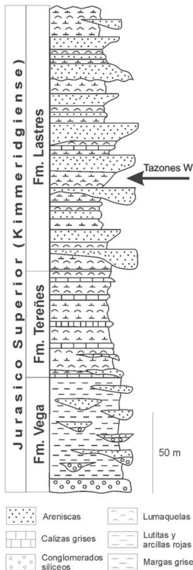
Fig. 2.- Columna estratigráfica del Jurásico Superior en la zona de Tazones.
