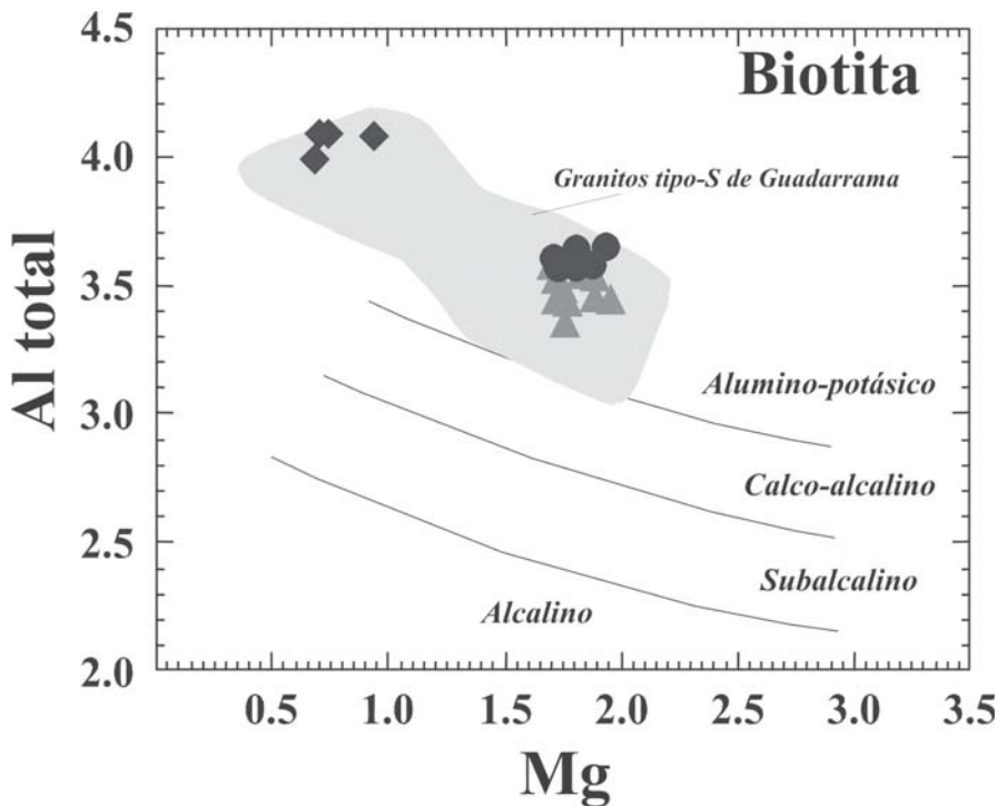
Fig. 1.- Diagrama Al_{tot} - Mg de clasificación química de biotitas (Nachit et al. , 1985). Los símbolos corresponden con: ●, biotitas de Aldeanueva; ▲, biotitas de Peraleda; y ◆, biotitas de Belvís. Se muestra también el campo composicional de biotitas de granitos peraluminicos de tipo-S de la Sierra de Guadarrama (Villaseca y Barbero, 1994).
