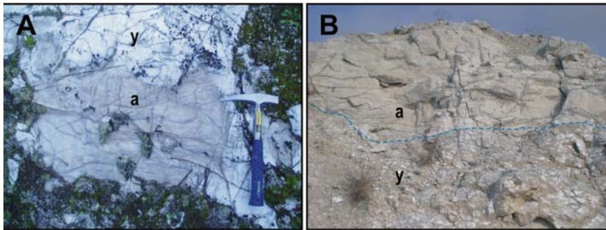
Fig. 3.- Masas anhidriticas residuales entre yeso secundario microcristalino (procente de la hidratación en superficie de la anhidrita). A. Formación de Yesos de Beuda (Maià de Montcal-Beuda, Girona). B. Formación de Yesos de Ódena (Ódena, Barcelona); el montículo tiene una altura de 4 m. a, anhidrita; y, yeso.
