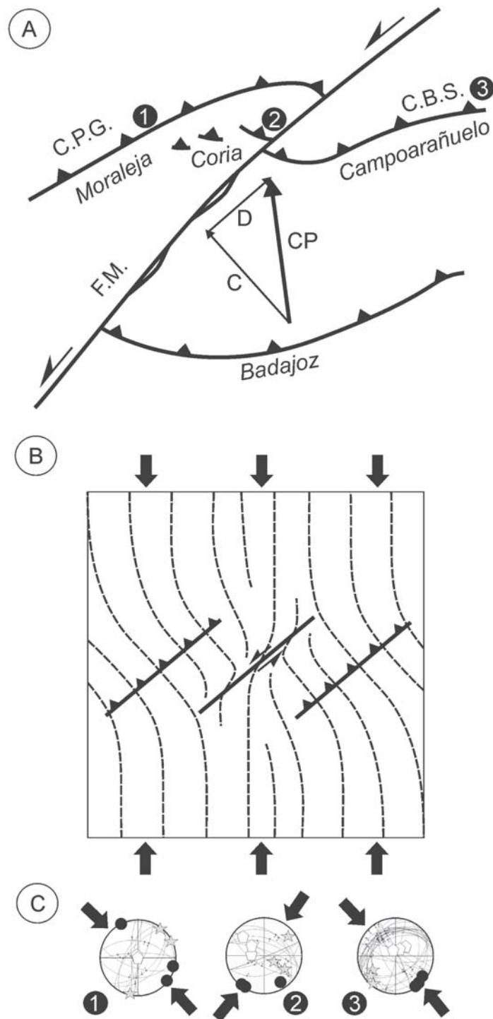
Fig. 3.- A) Modelo propuesto para la partición de la deformación cenozoica en el Sistema Central. CP dirección de convergencia Iberia-África hasta el Mioceno. C thrusting componente de los cabalgamientos. D vector compatible con el movimiento de la falla de Messejana. Las cuencas cenozoicas asociadas aparecen en cursiva. B) Trayectorias teóricas de los paleoesfuerzos ( s_{hmax} ) asociados al proceso de partición de la deformación. C) Estaciones «tipo» de poblaciones de fallas cenozoicas. Están localizadas en A) y las soluciones tensoriales obtenidas (todas compresivas). Negro, \sigma_1 . Gris, \sigma_2 . Blanco, \sigma_3 .
