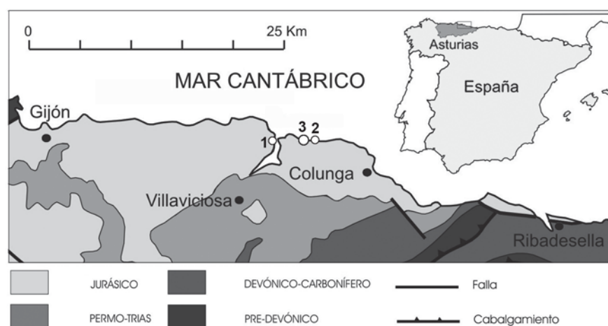
Fig. 1.- Situación geográfica y geológica de los yacimientos con restos de plesiosaurios del Jurásico Inferior de Asturias. 1: El Puntal-Tazones (Schulz, 1858), 2: Santa Mera (Bardet et al. , 2008a), 3: Villar (este trabajo). Modificada de Bardet et al. (2008a).
