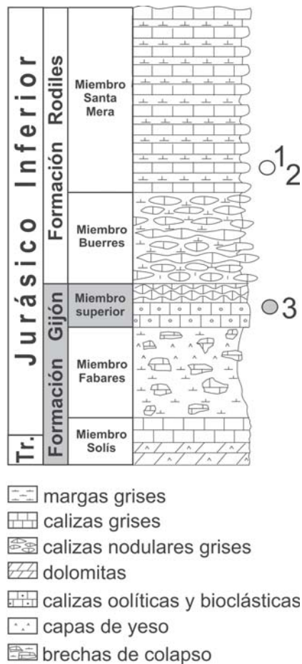
Fig. 2.- Situación estratigráfica de los yacimientos con restos de plesiosaurios del Jurásico Inferior de Asturias. 1: El Puntal-Tazonos (Schulz, 1858), 2: Santa Mera (Bardet et al. , 2008a), 3: Villar (este trabajo). Modificada de Bardet et al. (2008a).
