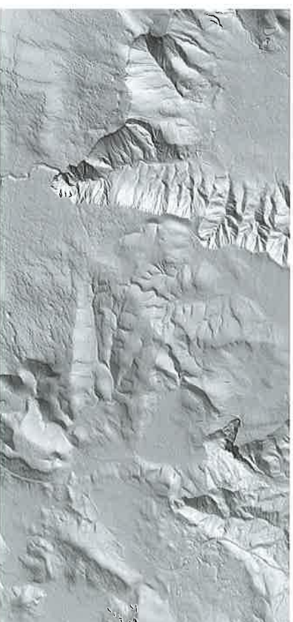
Figura 6. MDT LIDAR del karst de Santiago-Gulbijo y los barrancos de Gulbijo y Déléica
